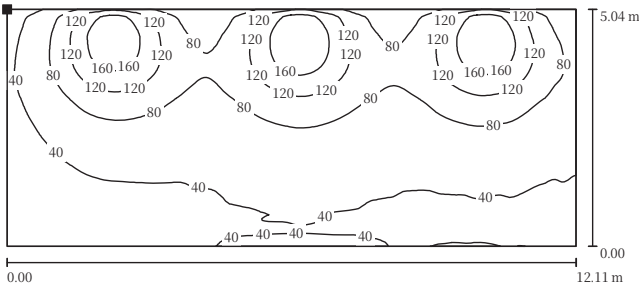
Values in Lux, Scale 1 : 87
