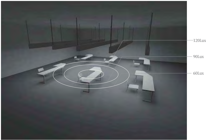
Values in Lux, Scale 1 : 200
